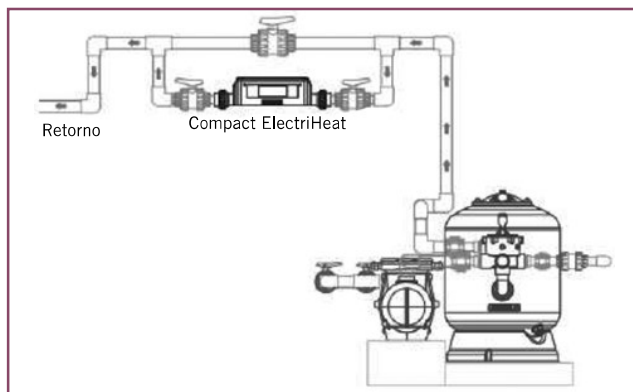
Correcta instalación - 1 intercambiador
