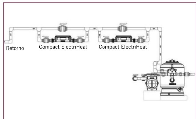
Correcta instalación - 2 o más intercambiadores
