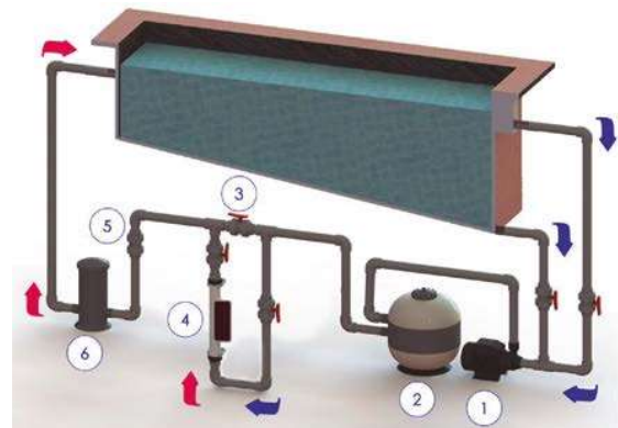
Instalación correcta de manera vertical.
