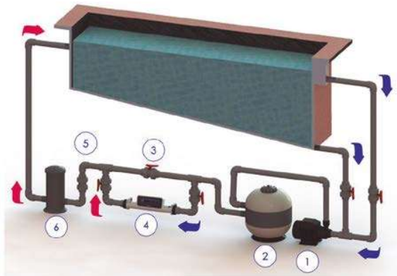
Instalación correcta de manera horizontal.
